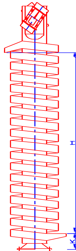
Alternativ udførelse med motorvibratorene placeret øverst.
